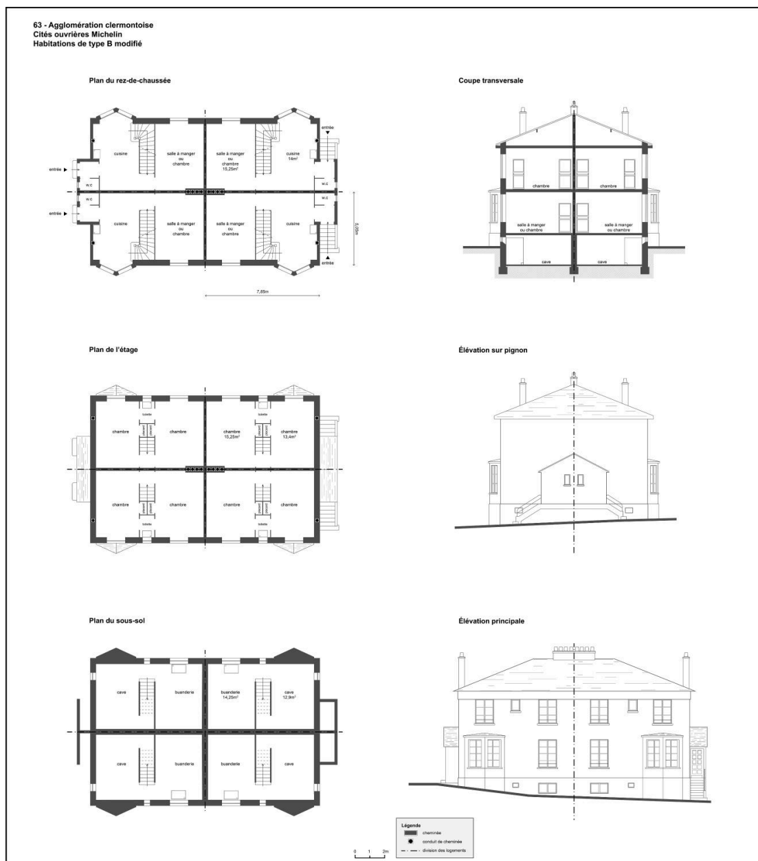
Plan des habitations de type B modifié.
