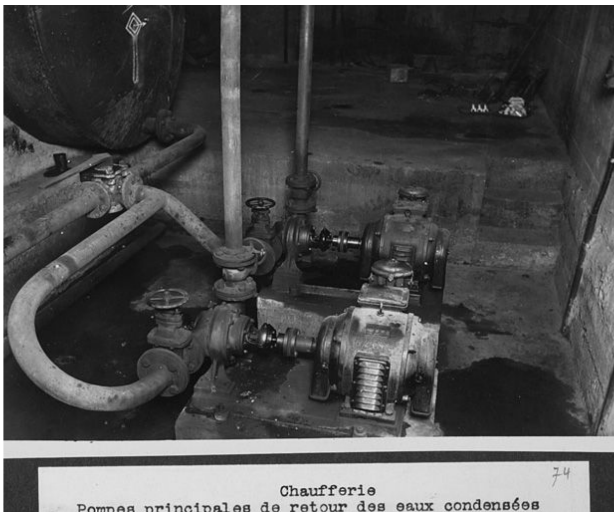
Chaufferie. Pompe principale de retour des eaux condensées. Photogr., vers 1960
