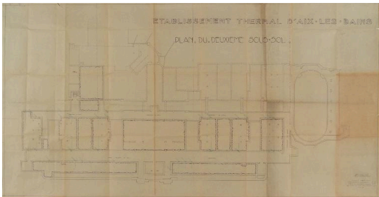
Plan du 2ème sous-sol
