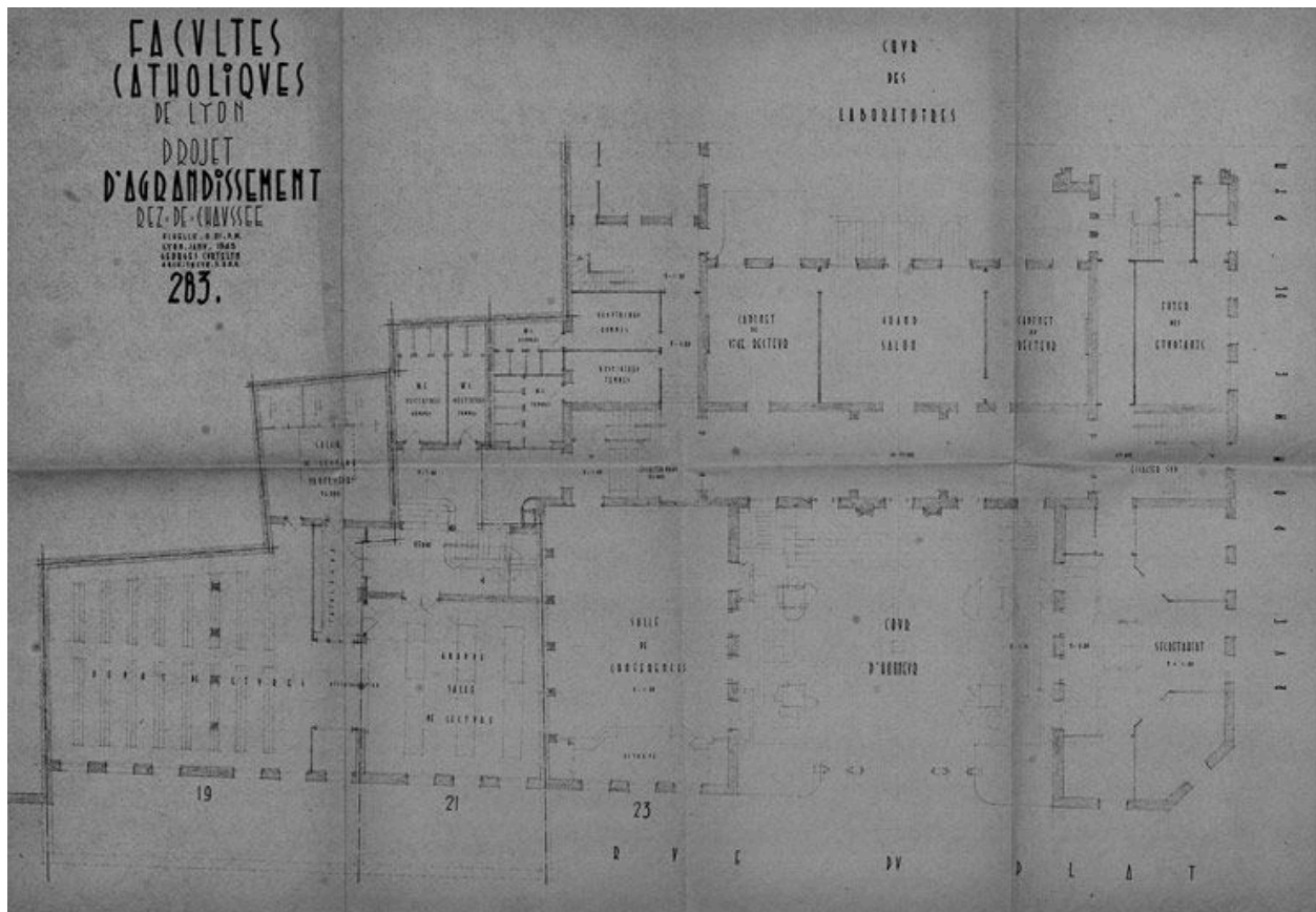
Plan, projet d'agrandissement du rez-de-chaussée, par G. Curtelin, 1943
