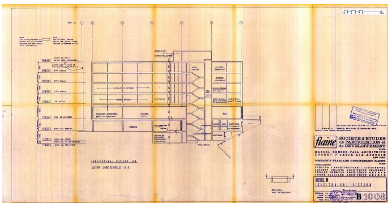
Hôtel B. Coupe longitudinale. Marcel Breuer architecte, Robert F. Gatje associé, 15 janvier 1962. Modification 9 mars 1962 (AC Arâches-la-Frasse)
