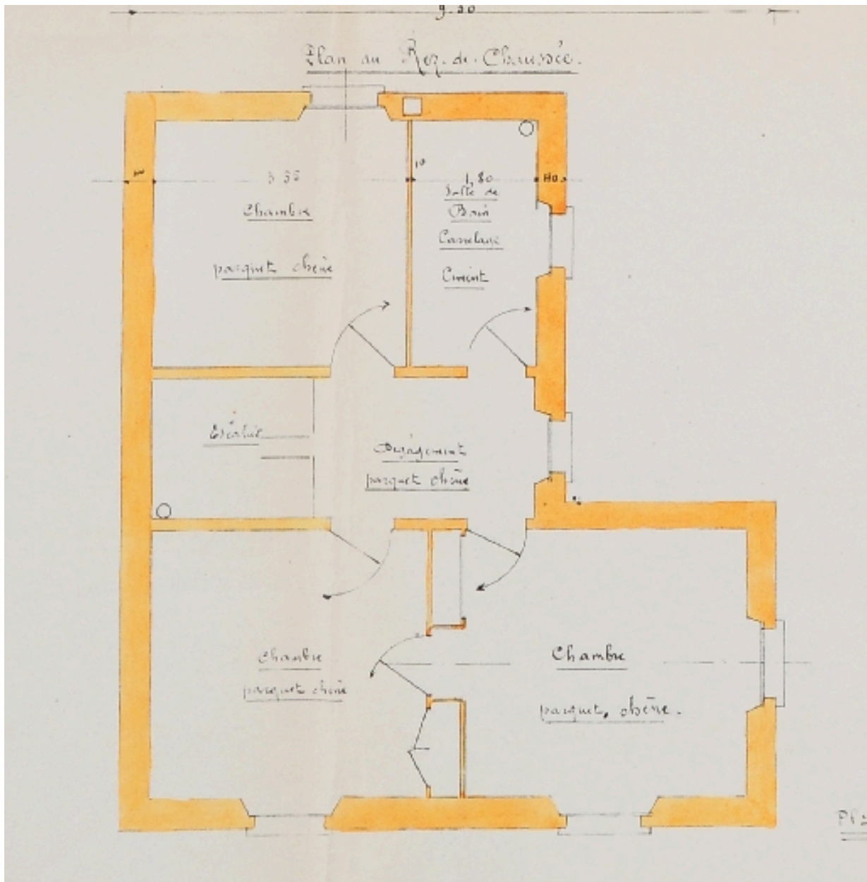
Plan de l'étage
