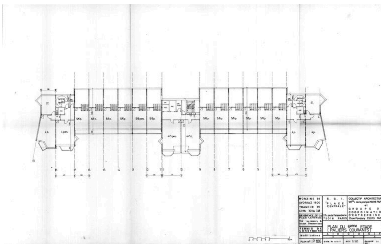
Plan du 6e étage (paliers courants) / Collectif architecture et groupe de coordination d'entreprise, 12 octobre 1977 (AC Morzine)
