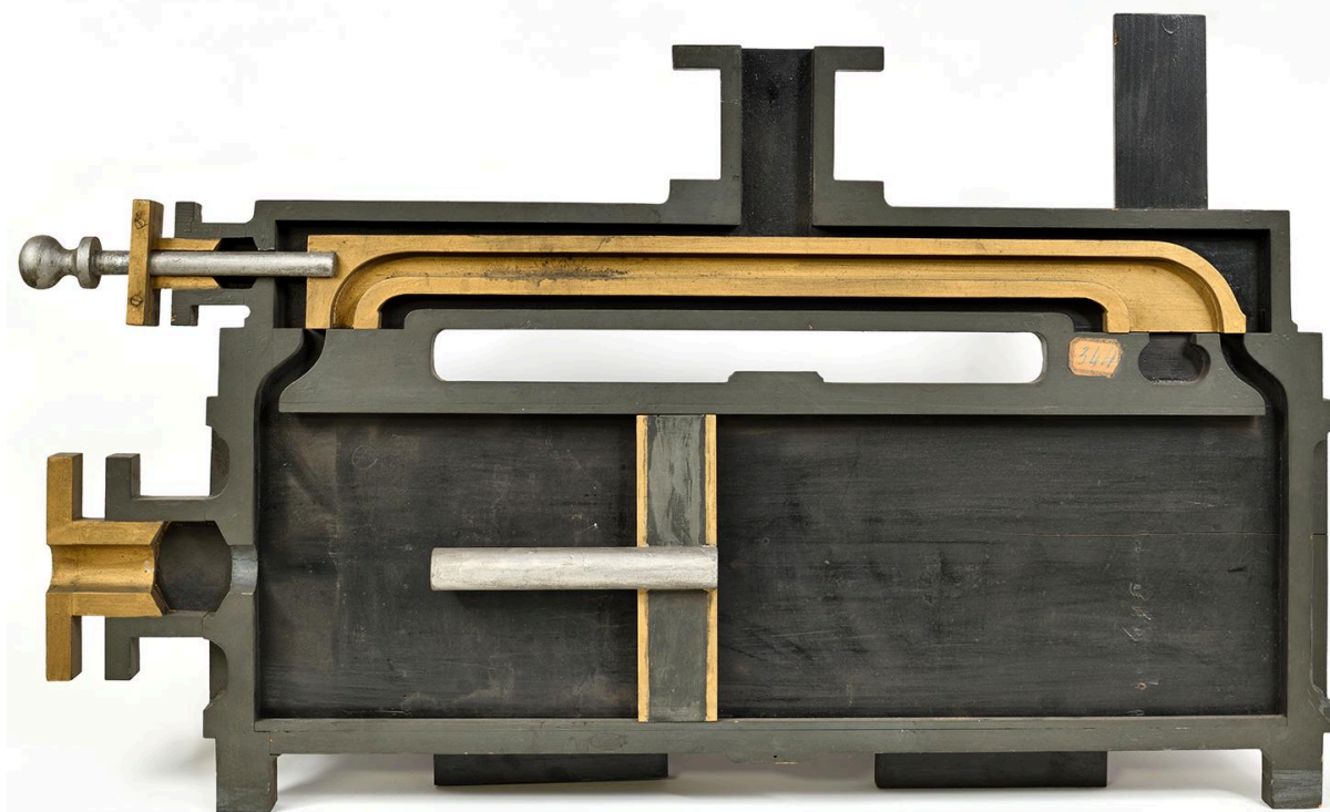
Maquette de piston
