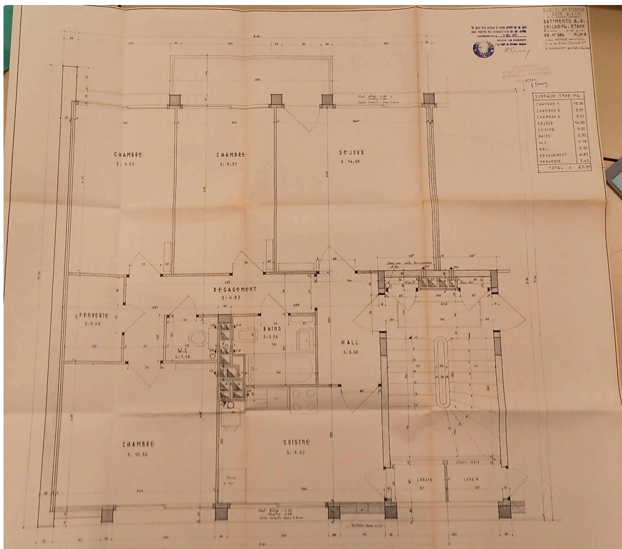
Plan d'un appartement à l'étage
