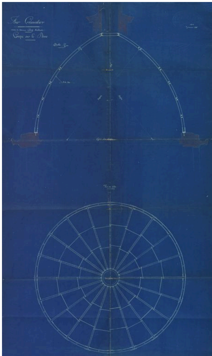
Dôme : coupe et plan, 8 janvier 1908
