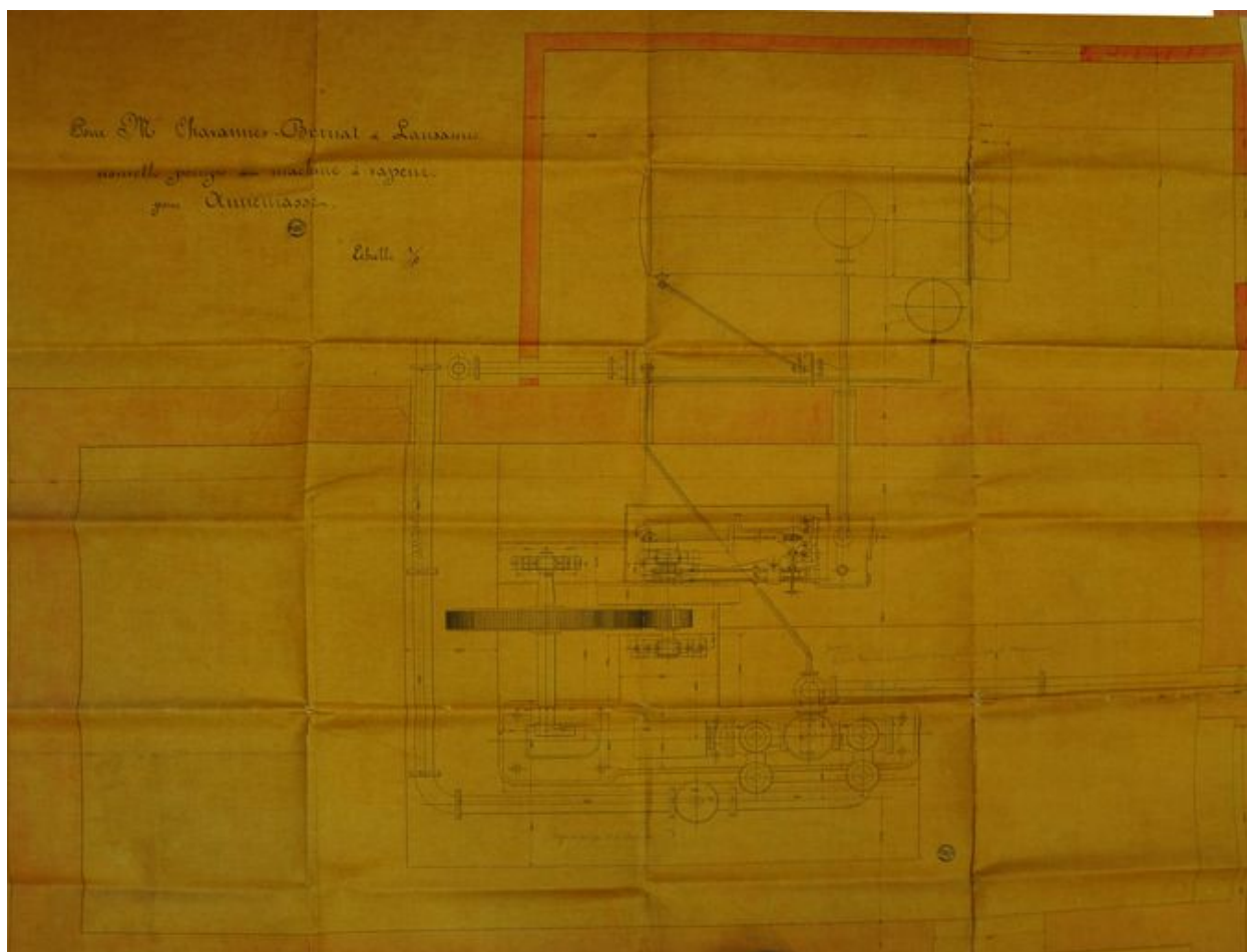
Coupe transversale de la machine hydraulique d'Annemasse. Plan. Archives municipales d'Annemasse © Archives municipales d'Annemasse. 36/36
