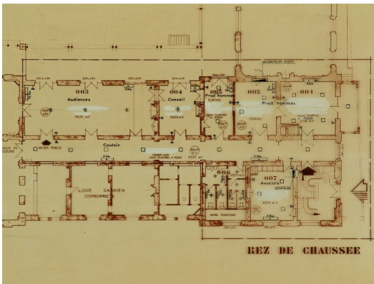
Plan du rez-de-chaussée du tribunal, aile nord du corps principal
