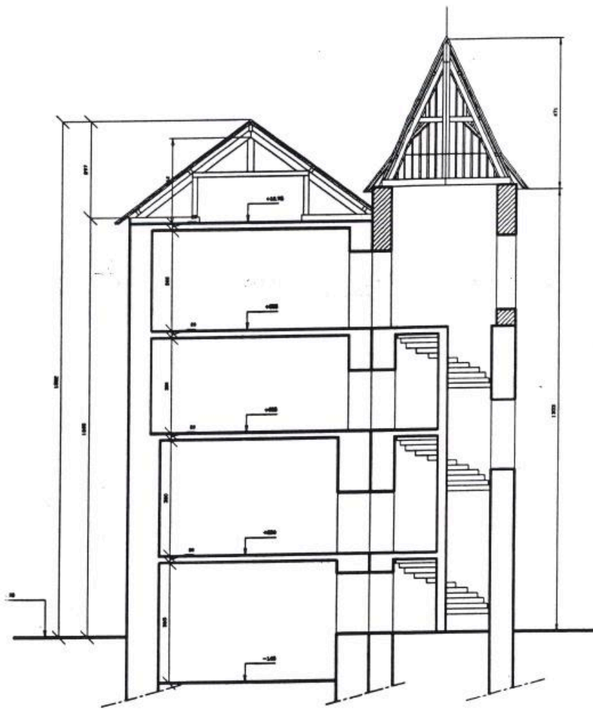
PROJET COUPE AA' ECH:1/100
