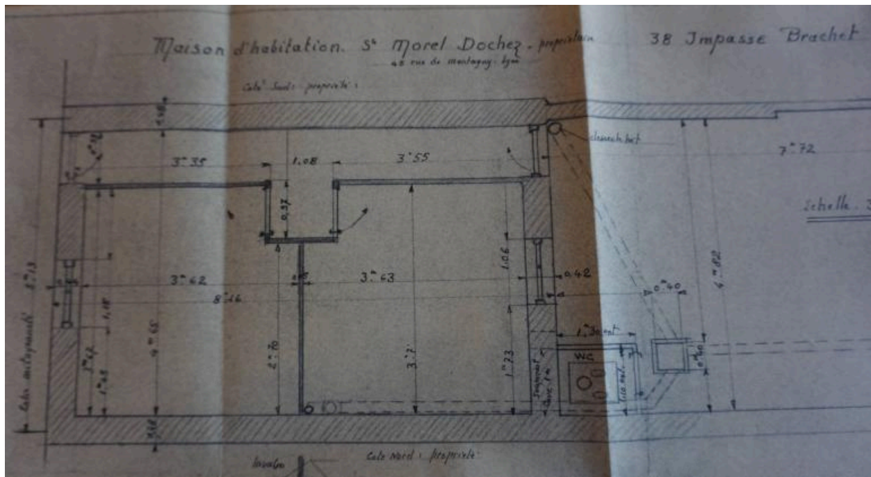
Plan maison d'habitation de la Société Morel & Dochez - 38 impasse Brachet (AC Lyon, 1097W/619)
