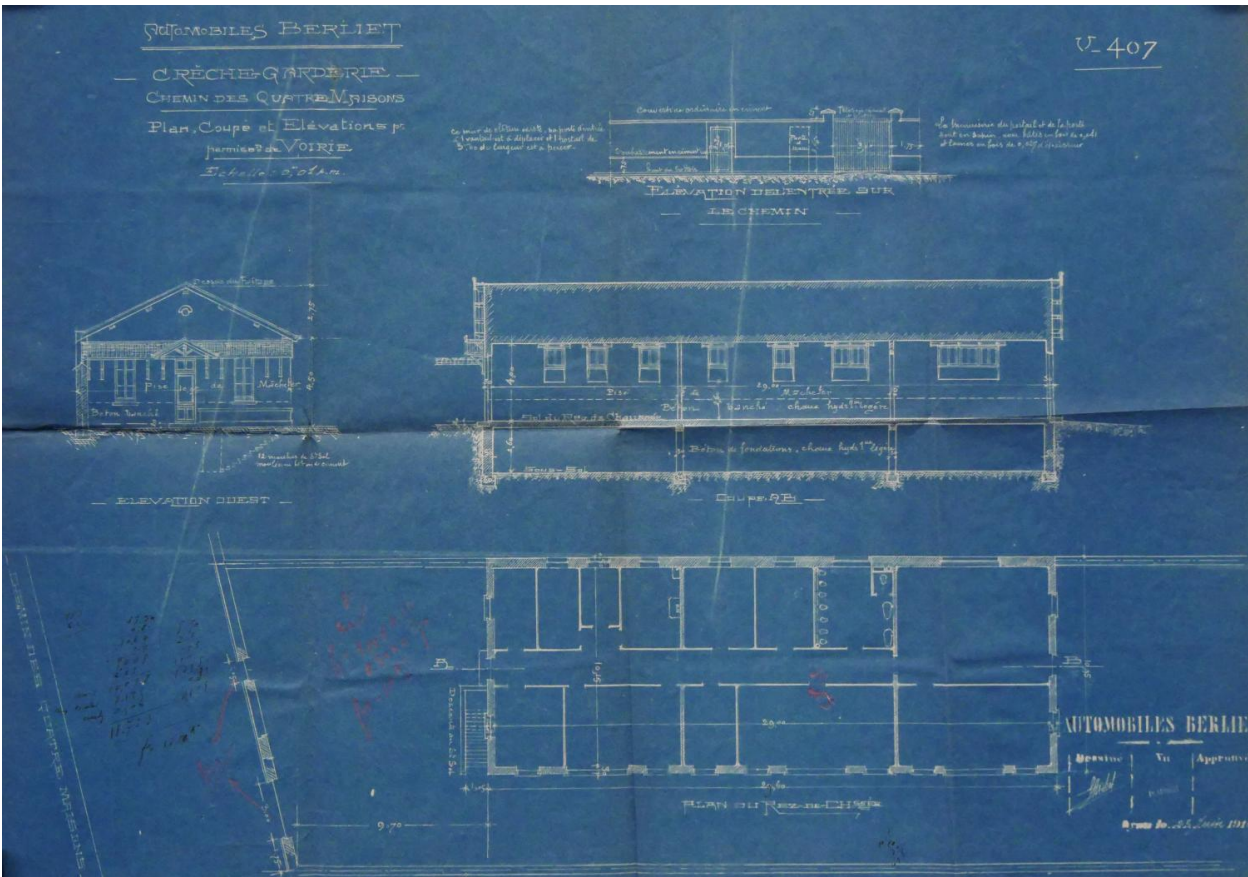
Plans élévation 1916, crèche garderie usine Berliet rue des quatre maisons, Lyon 8e (ACL314w575-135)
