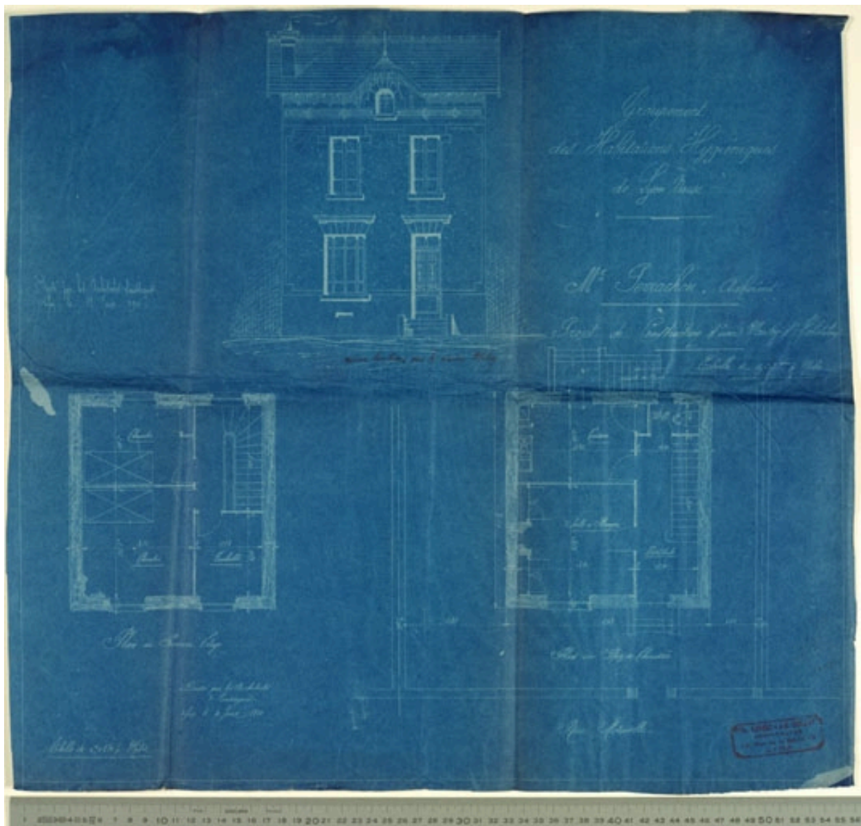
314 WP 1910 permis 527, plans, façade d'une maison individuelle au 24 rue Littré
