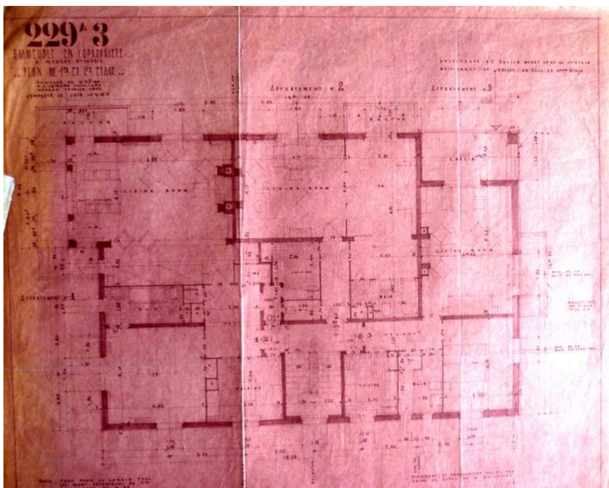
Plan du 1er et 2e étage. Henry Jacques Le Même, janvier-juin 1945 (AD Haute-Savoie. 142J 939)
