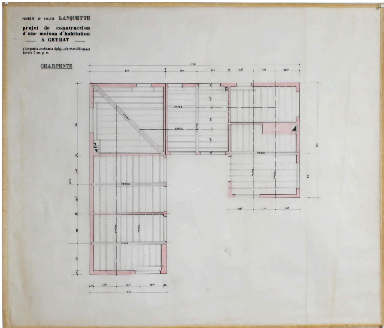
Ceyrat, la maison L., plan de la charpente, 24 juin 1964, Paul Lanquette architecte (archives privées famille Lanquette).
