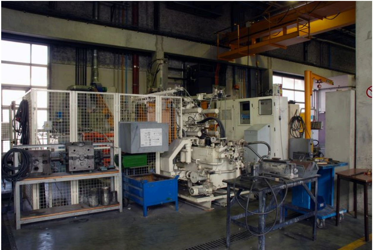
Machine à moulage sous pression : IDRA PRESSE
