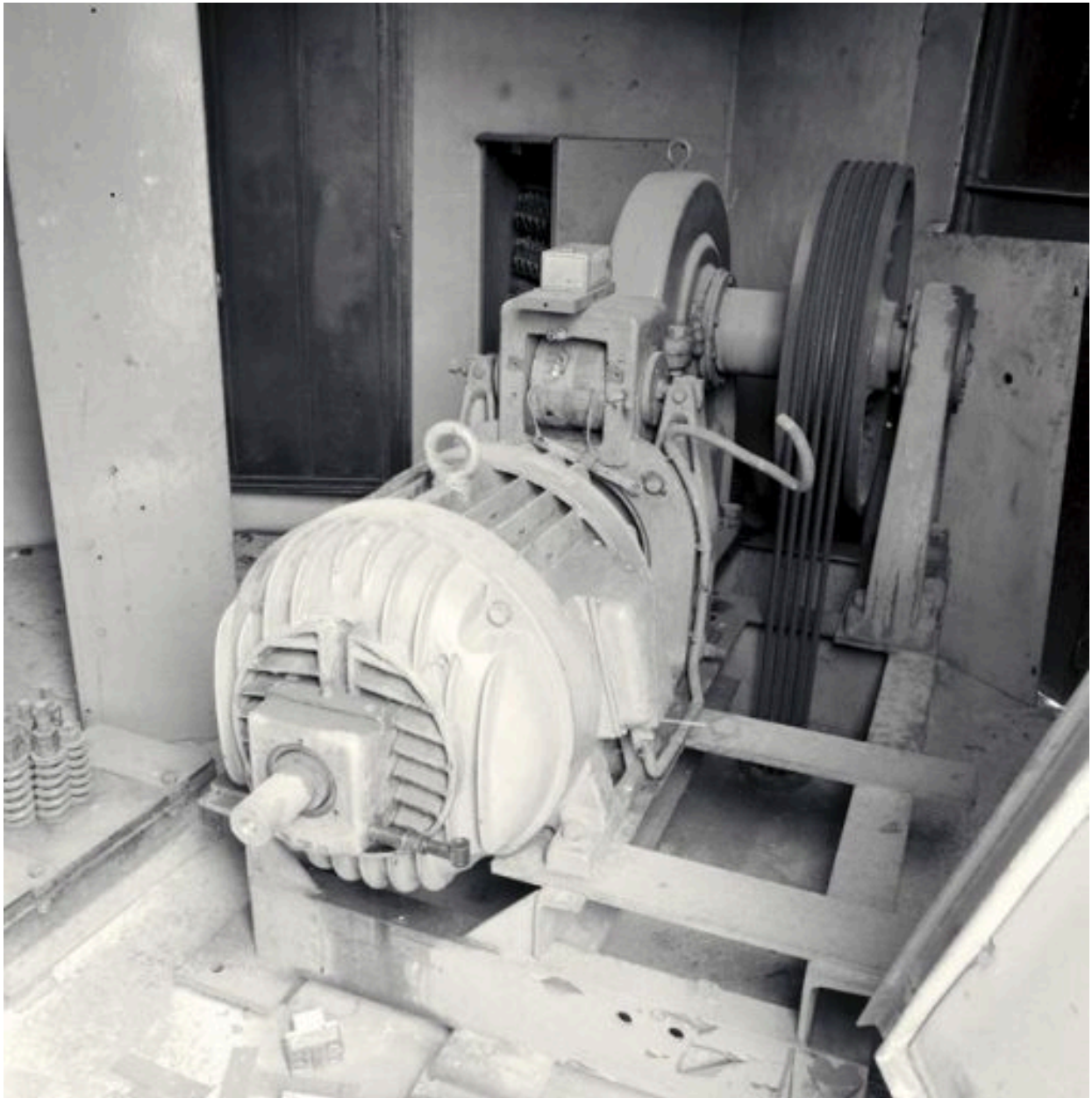
La machinerie d'ascenseur OTIS 346 JY, sur le toit terrasse
