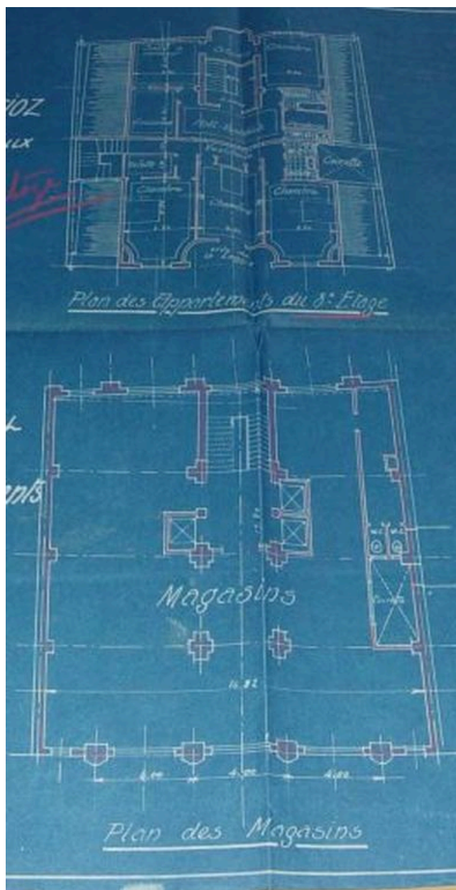
Plan du 8e étage et plan des magasins
