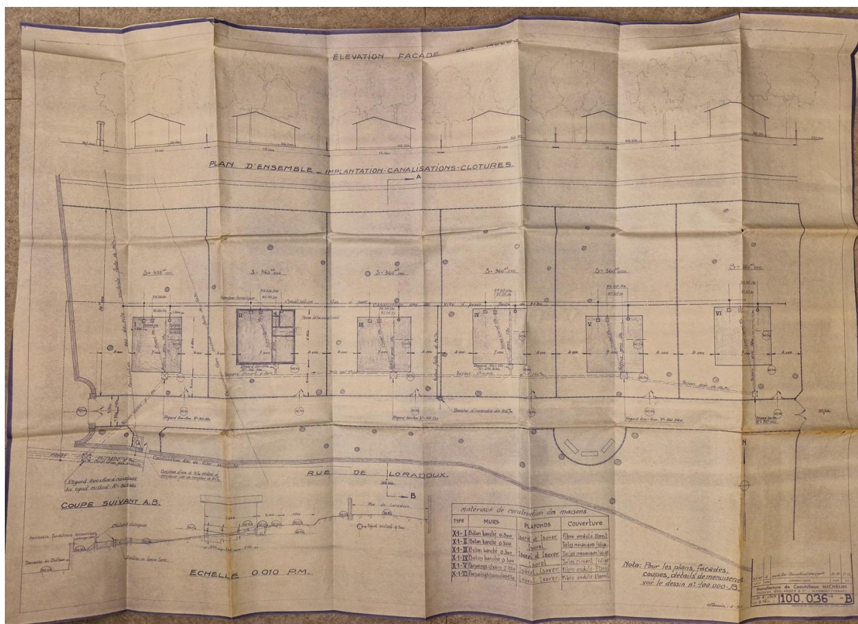
Projet de construction de six maisons individuelles de type X1 : plan d'implantation, coupe sur le terrain et ensemble des élévations, 1949.
