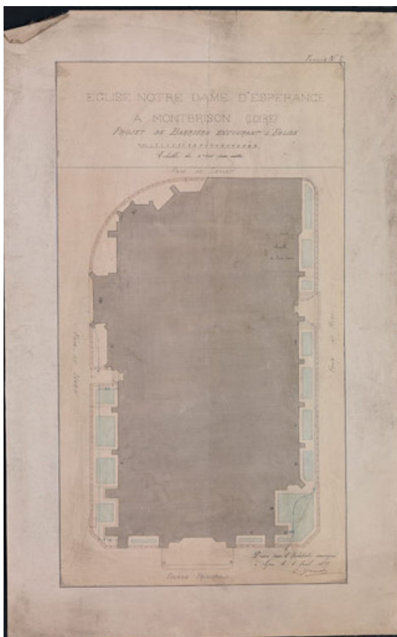
Eglise Notre Dame d'Espérance à Montbrison. (Loire). Projet de barrière entourant l'église. Feuille n°2.
