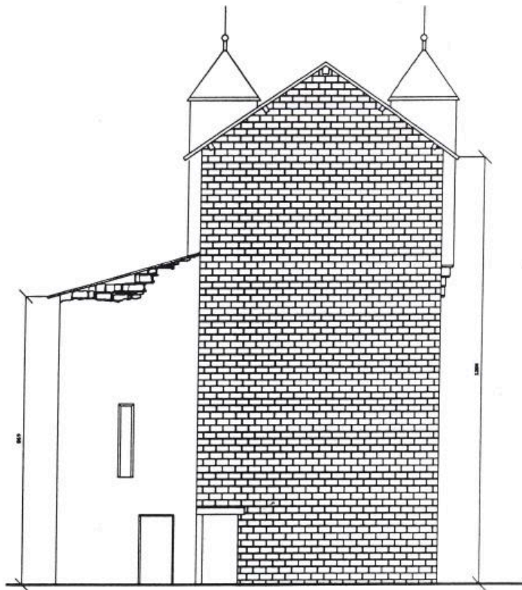
ETAT DES LIEUX FACADE EST ECH:1/100
