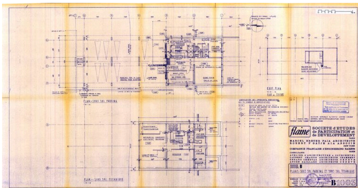
Hôtel B. Plan du sous-sol. Marcel Breuer architecte, Robert F. Gatje associé, 15 janvier 1962. Modification 9 mars 1962 (AC Arâches-la-Frasse)
