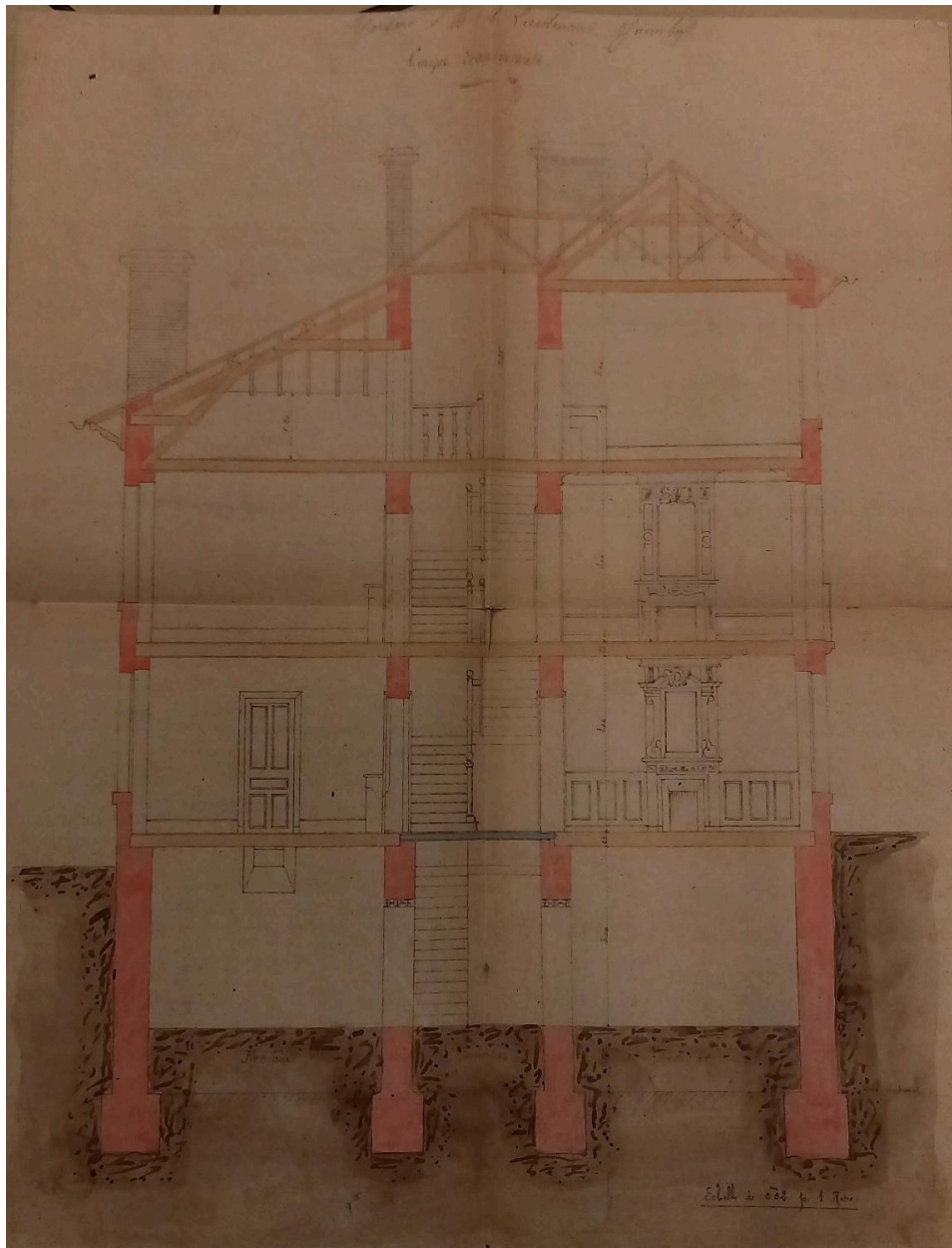
coupe de la maison, 41 avenue d'Italie
