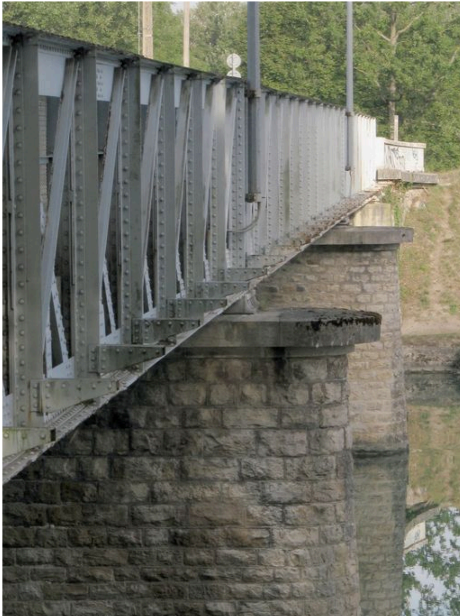
Vue partielle, de côté, tablier et haut des piles, face amont (depuis la rive gauche)
