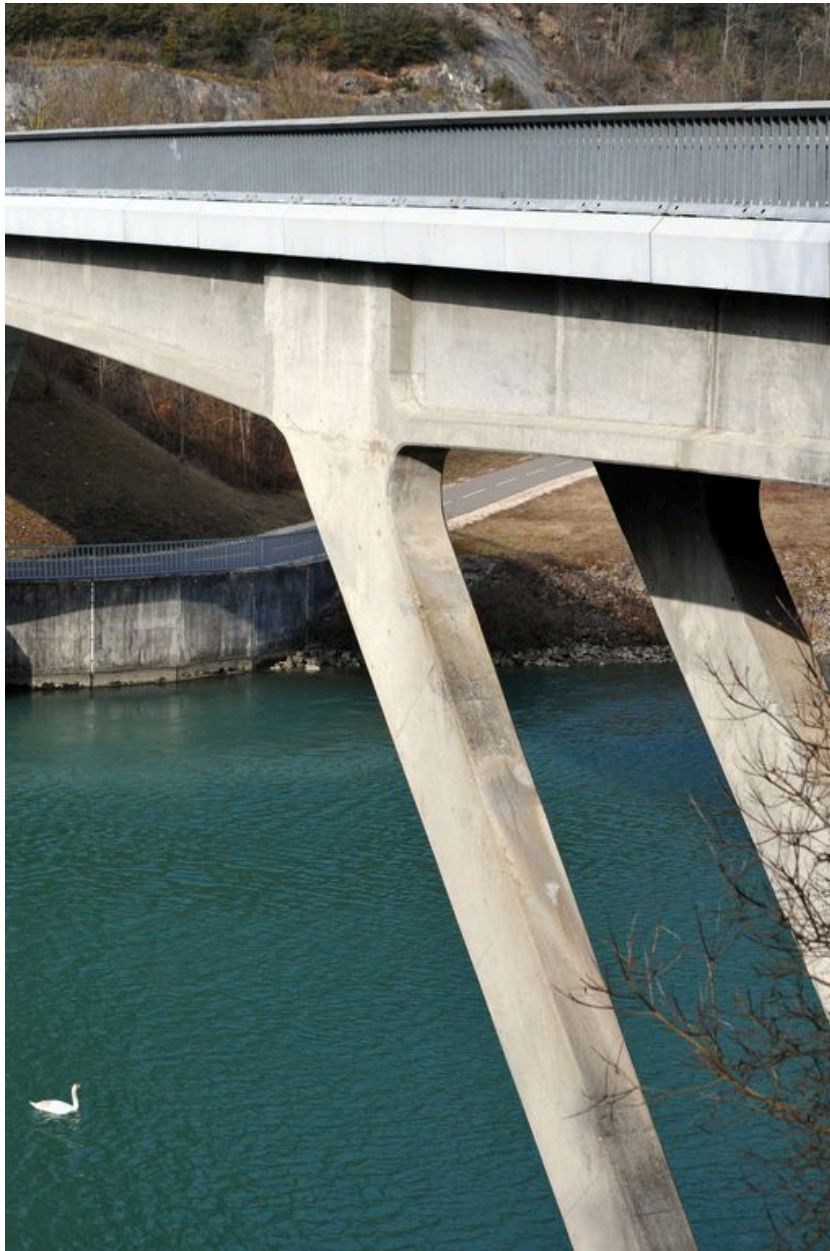
Béquille gauche, face aval, vue partielle : jonction d'un des appareils d'appui avec le tablier (depuis la rive gauche)
