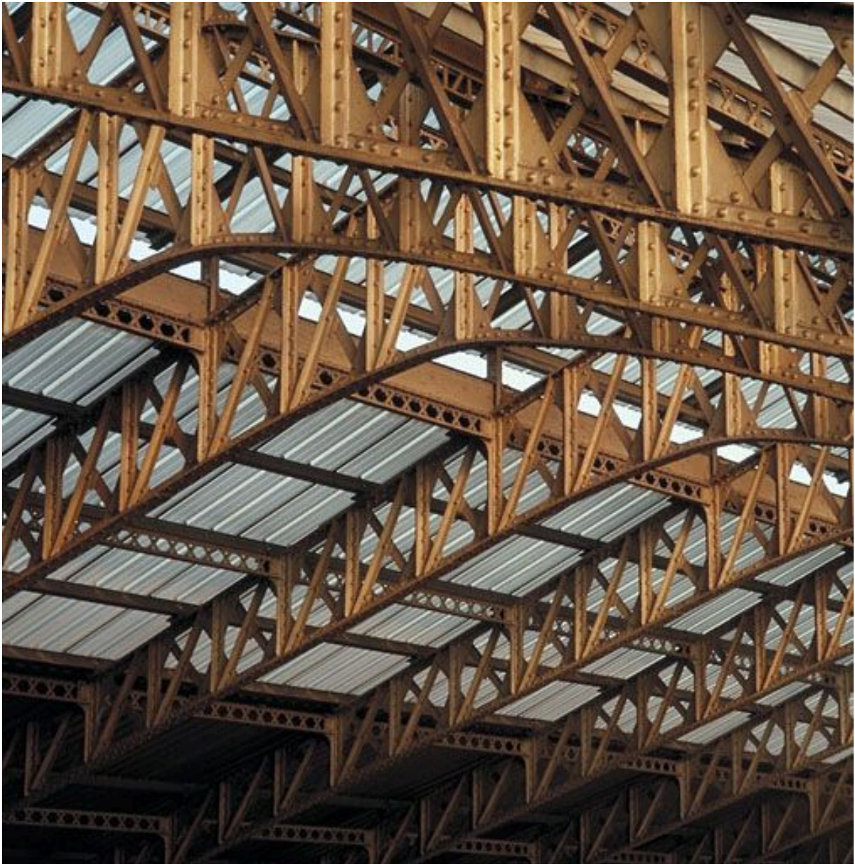
Halle Saint-Etienne : détail de la charpente métallique
