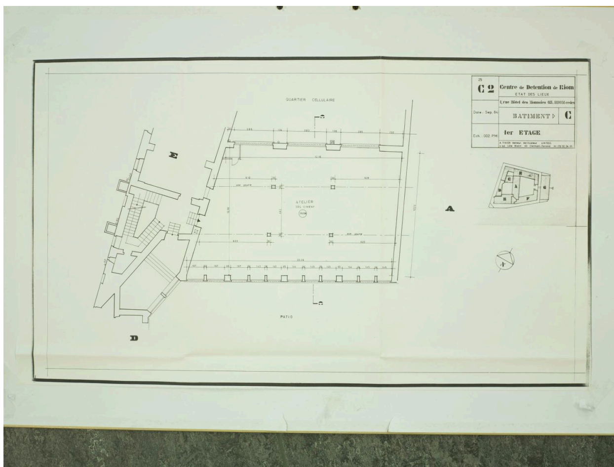
Bâtiment C, plan, 1er étage, éch. 002 p.m. État des lieux, septembre 1984.
