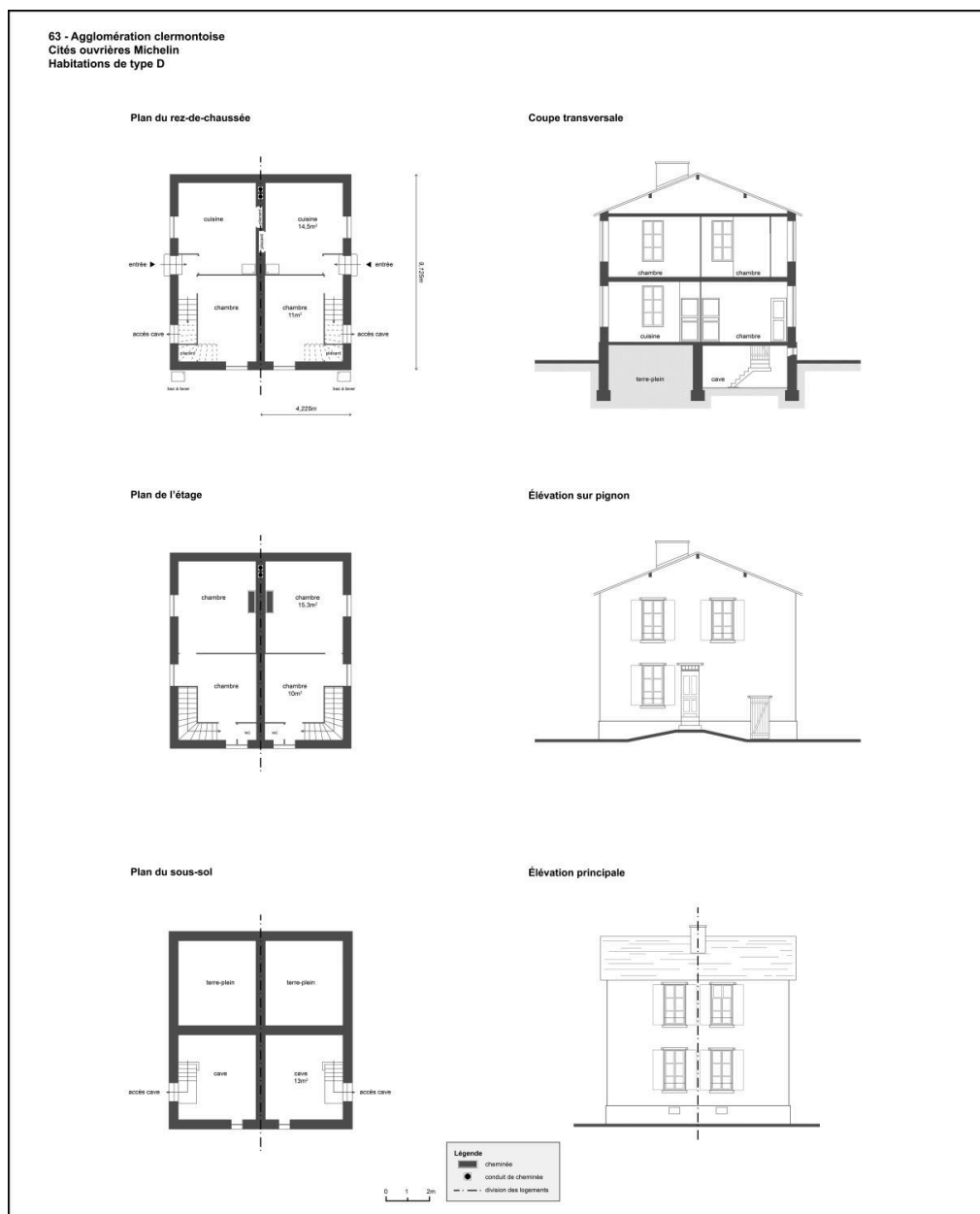
Plan des habitations de type D.
