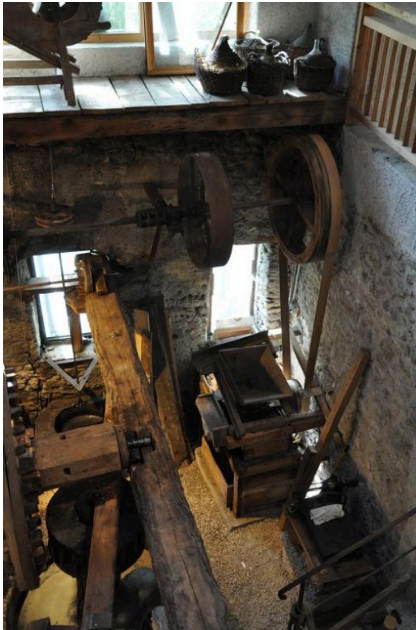
Mécanismes du moulin à huile.
