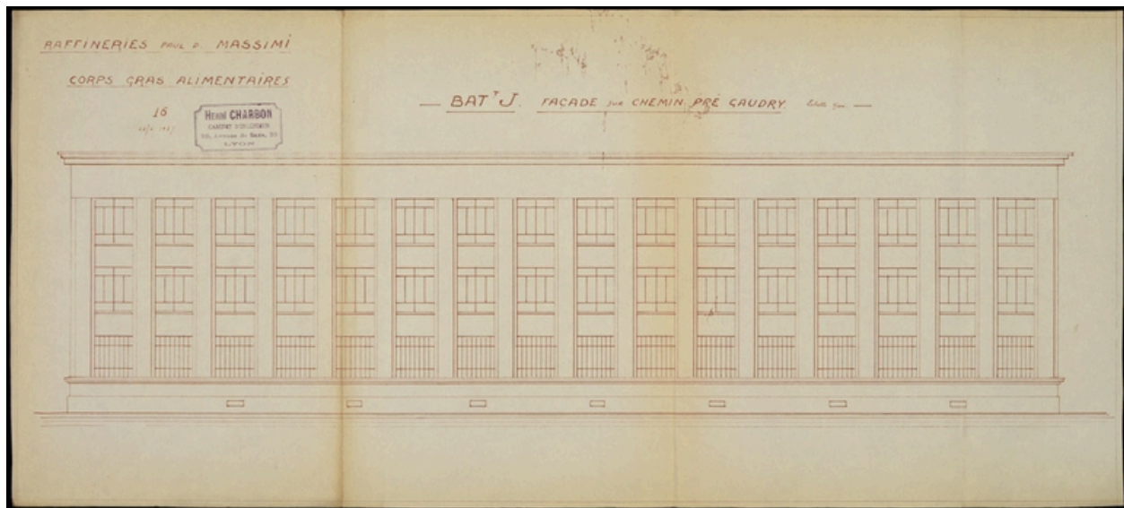
Façade bâtiment J (ACL : 344 WP 1937-414., 1937, Charbon ingénieur)
