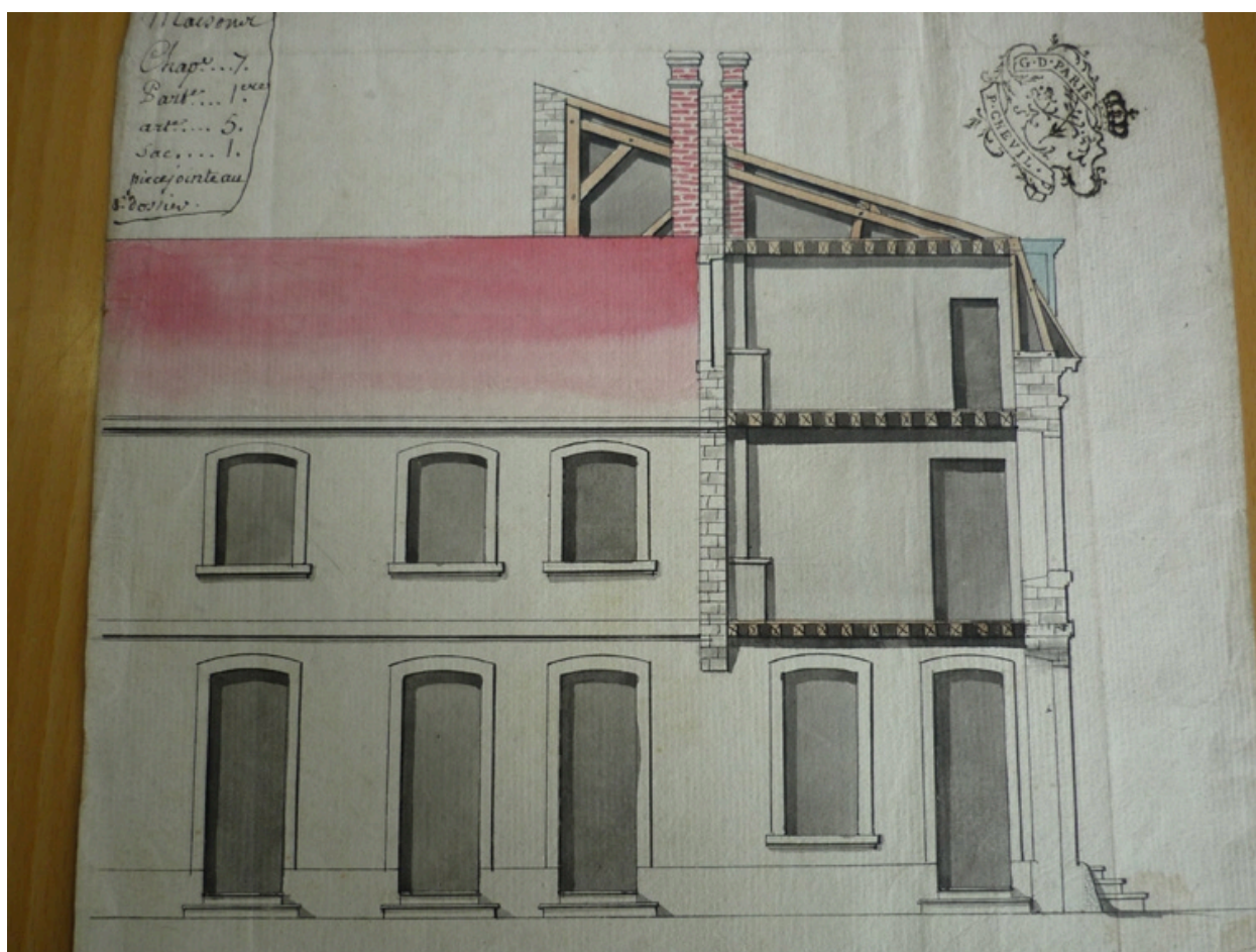
Elévation et coupe du corps de logis du grenier à sel, 17 mai 1740 (détail). Plan AC Lyon. Fonds des HCL ; B421
