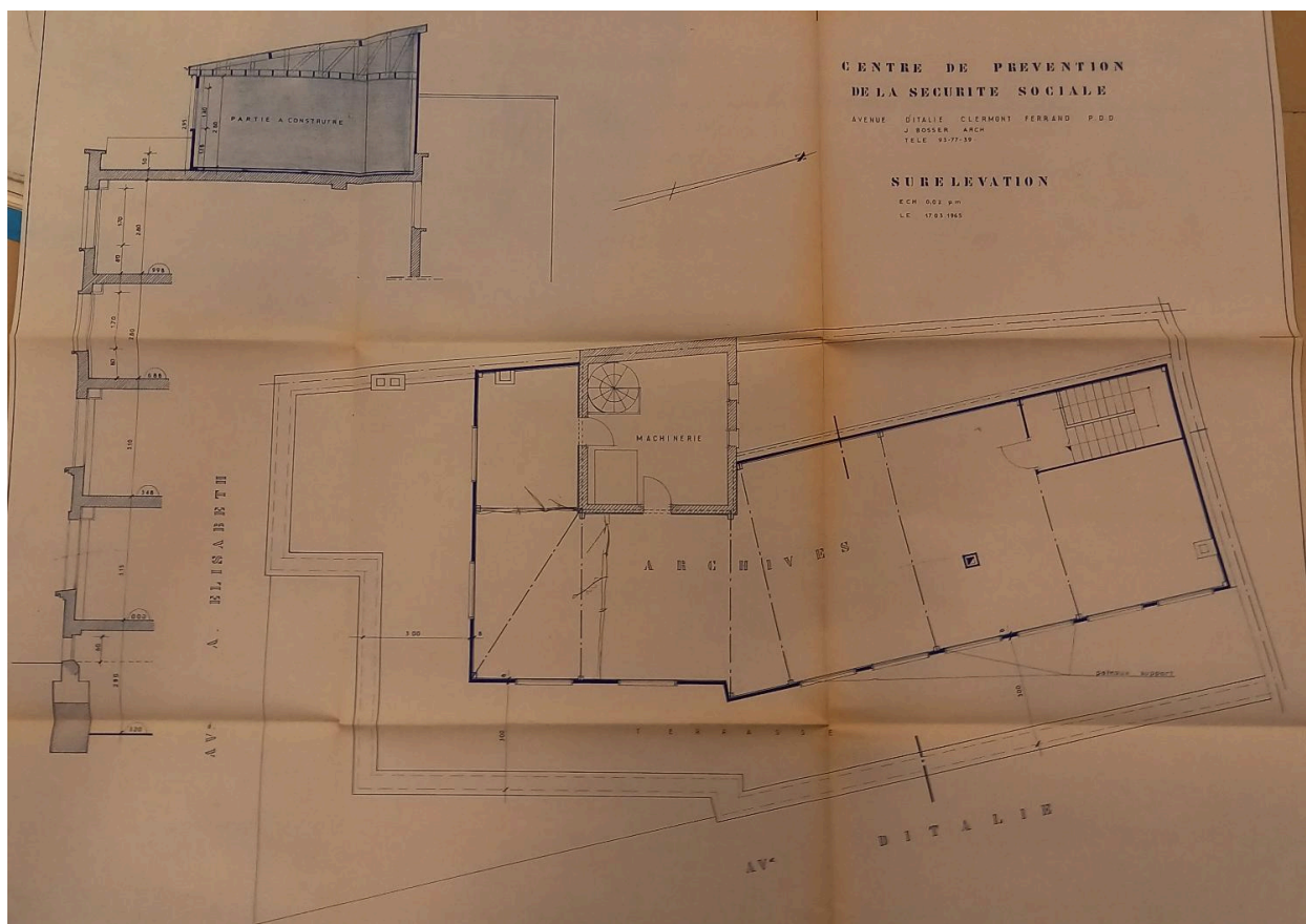
Coupe et plan de l'étage en surélévation, 50 avenue d'Italie
