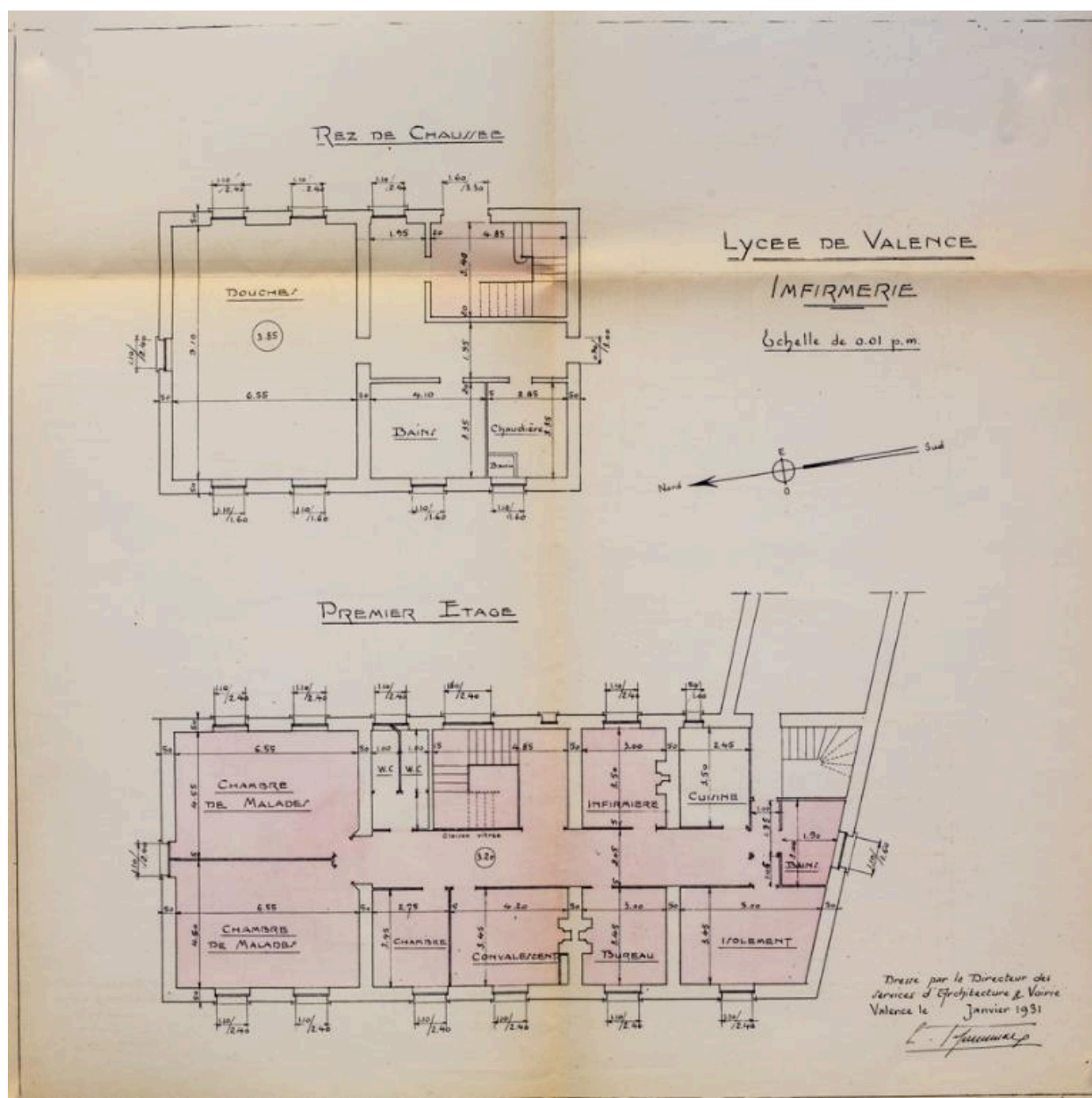
Plan. Infirmerie. Sous-sol, premier étage, 1931
