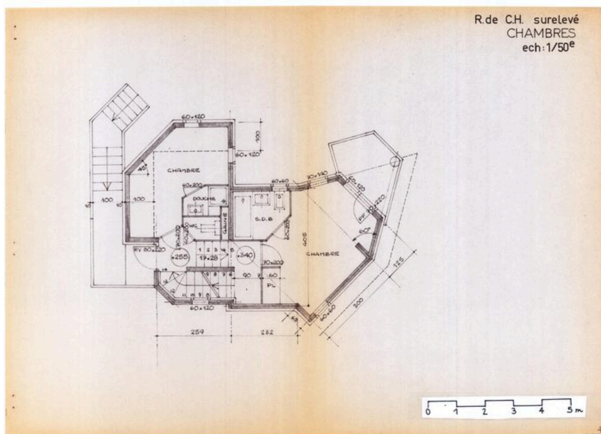
Plan du rez-de-chaussée surélevé / J. Labro, 1979 (A. privées J. Labro)
