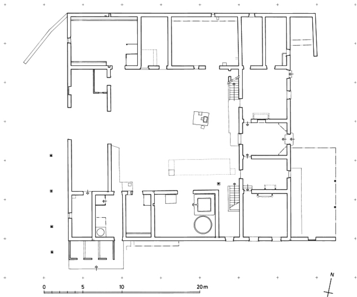
Plan du rez-de-chaussée. Relevé expédié et schématique.
