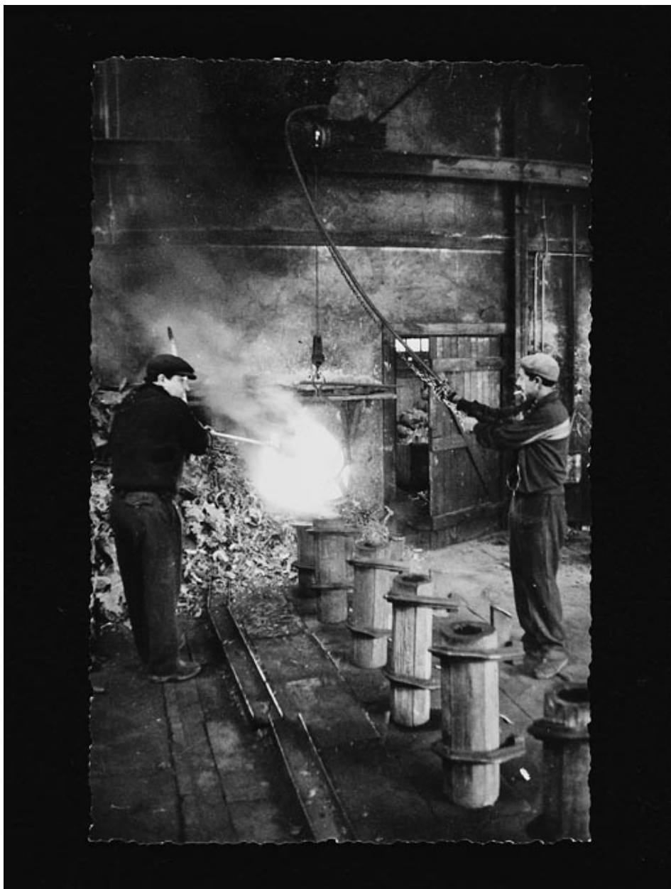
Cuivre en fusion versé dans des lingotières, atelier fonderie en activité jusqu'en 1960
