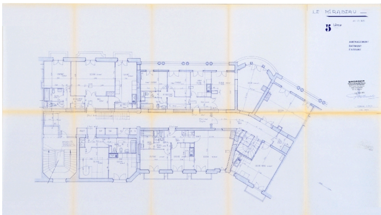
Plan d'aménagement du 4e étage, 1979
