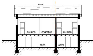
Coupe longitudinale
