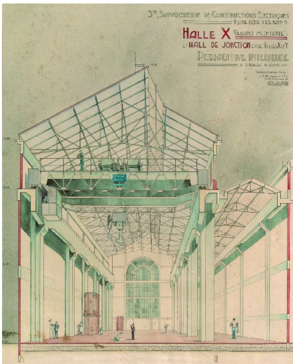
Perspective sur la halle X et le hall de jonction XY
