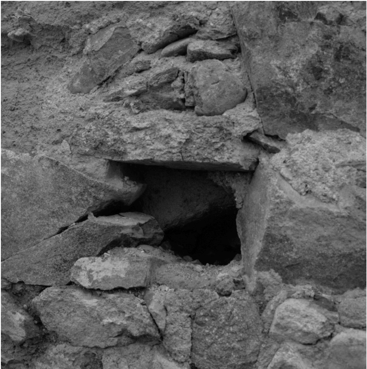
Façade sur jardin du corps de galerie après décroûtage, partie centrale en pisé du corps primitif : détail d'un trou de calage de banche pour la mise en oeuvre du pisé.
