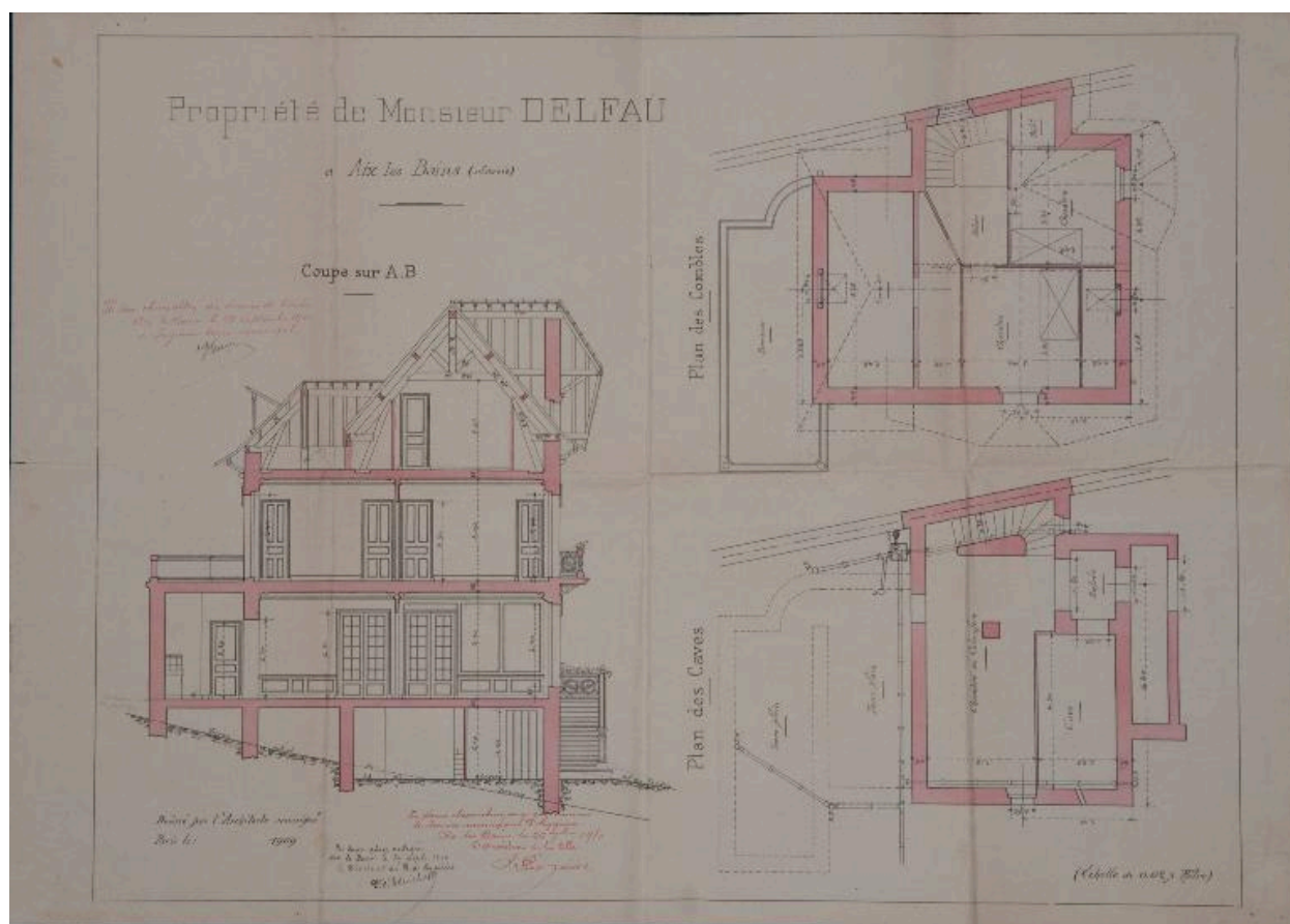
Coupe et plans des caves et combles, 1909
