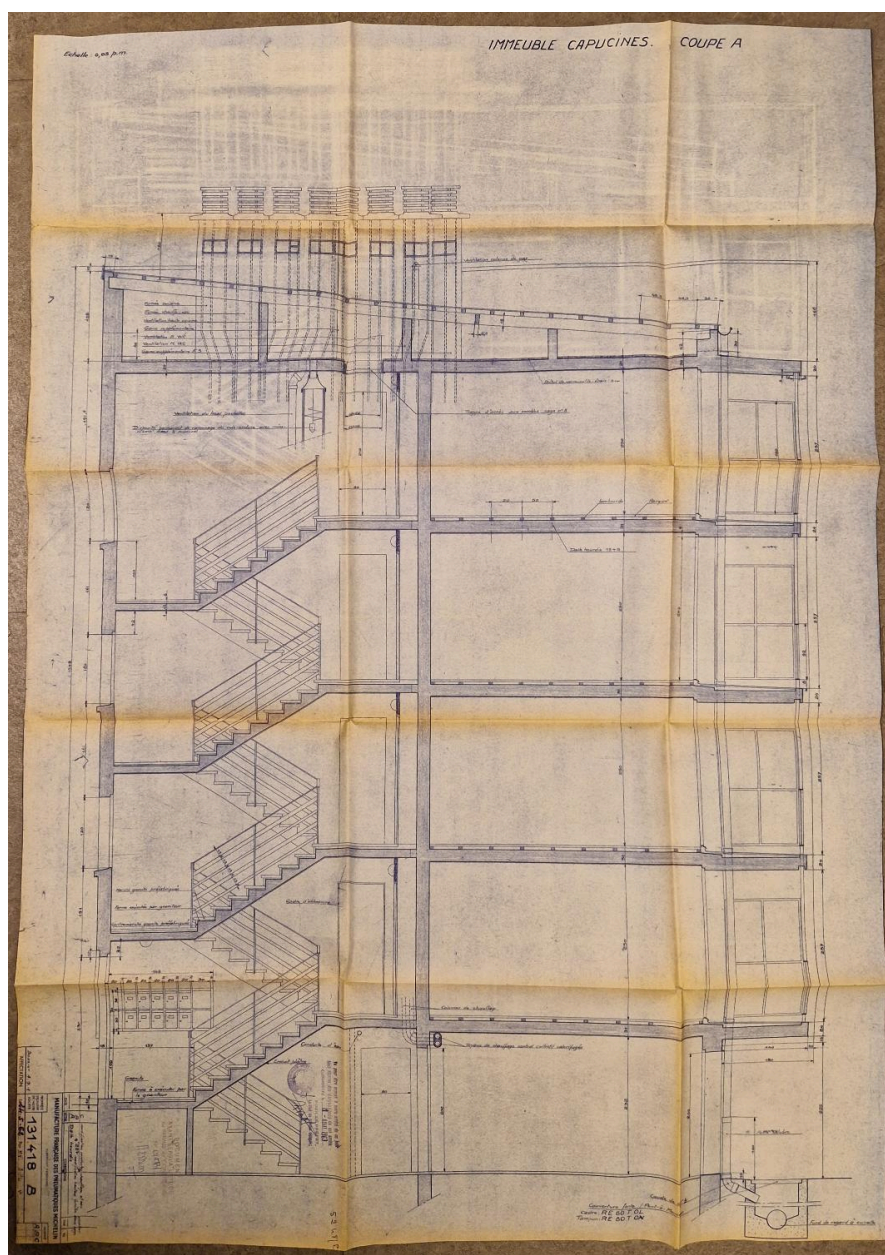
Projet des immeubles "les Capucines" à Lachaux : coupe transversale, 1962.
