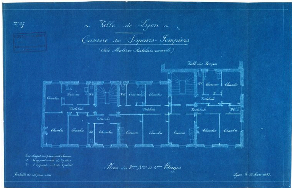
Plan des 2e, 3e et 4e étages, 13 mars 1923
