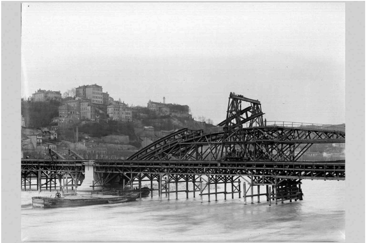
La construction du pont de la Boucle. La construction de la 1ère arche supérieure. Photogr., [1903] (Arch. mun. Lyon. 15 Ph 1824)
