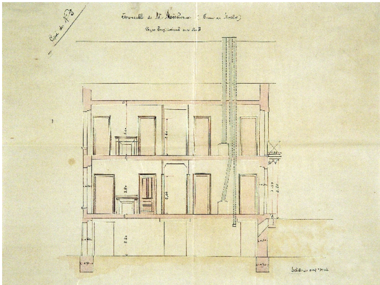
Coupe, 1893
