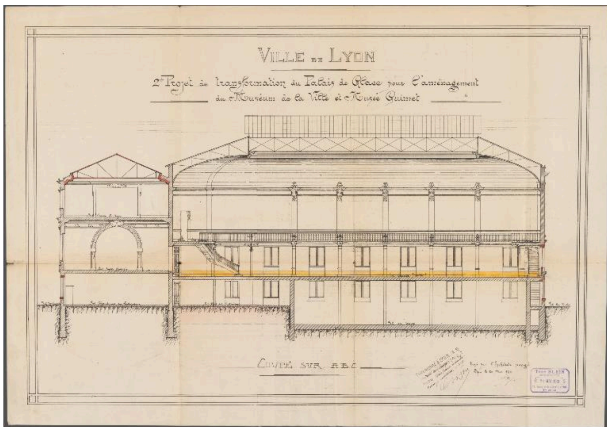
Deuxième projet de transformation du Palais de Glace pour l'aménagement du Muséum de la Ville et du Musée Guimet, coupe sur ABC (à gauche le boulevard, à droite la rue Boileau), Tony Blein architecte, 20 mai 1911. AC Lyon, 515 WP 6 2
