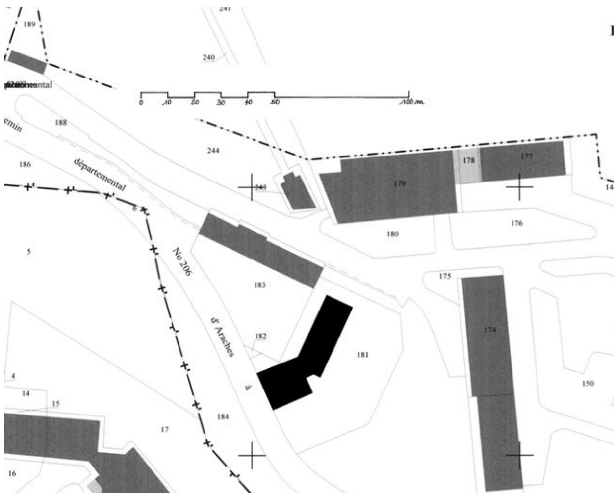
Plan masse, d'après le plan cadastral d'Arâches-la-Frasse, section CO1 183, 2006
